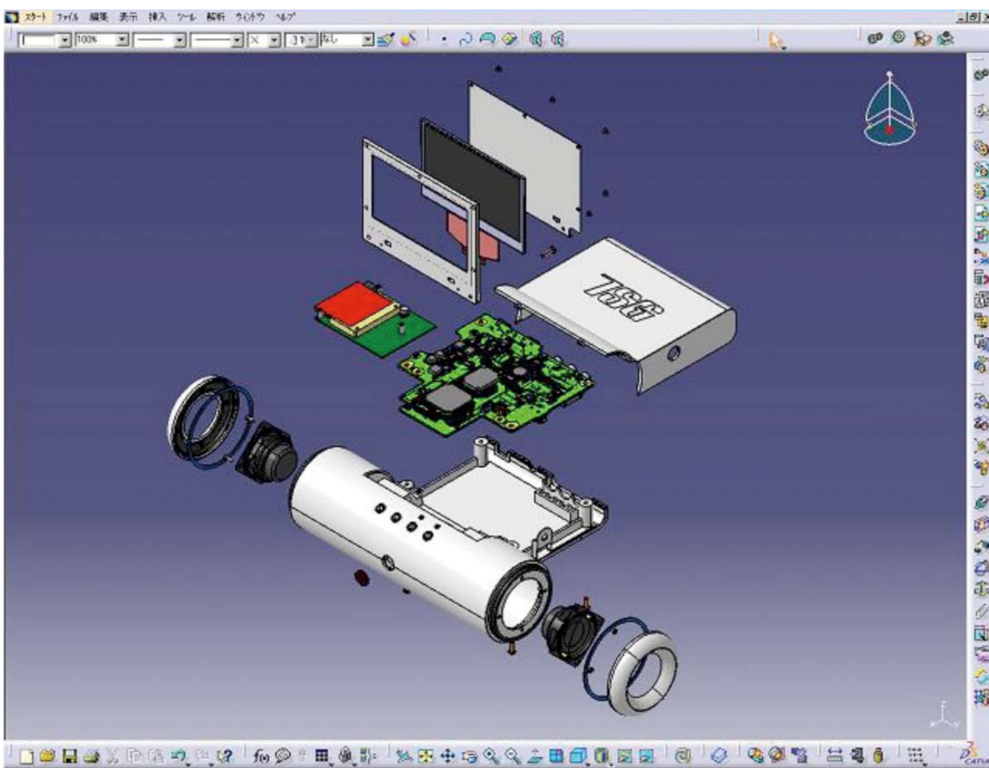
有機 EL ディスプレイ構造 (CATIA V5)
